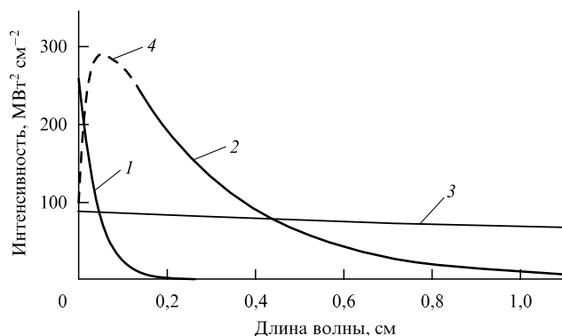
Рис. 3. Рассчитанное в диффузном приближении распределение интенсивности распространяющегося в ткани предстательной железы собаки излучения: 1 — Ho:YAG-лазера с длиной волны \lambda \approx 2,09 мкм, 2 — Nd:YAG-лазера с длиной волны \lambda \approx 1,064 мкм, 3 — интенсивность излучения Nd:YAG-лазера в отсутствие рассеяния, 4 — ожидаемая форма распределения интенсивности излучения в приповерхностном слое.
