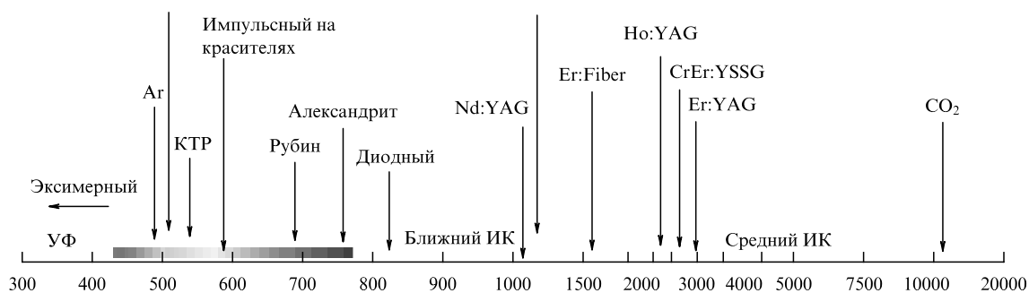
Рис. 1. Типы и длины волн излучения лазеров, применяющихся в медицинской практике.
